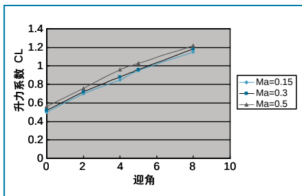
图8 不同来流速度下升力系数与迎角的关系图
