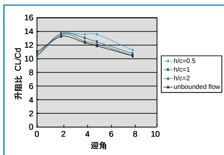
图13 不同飞行高度下升阻比与迎角的关系图
