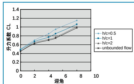
图11 不同飞行高度下升力系数与迎角的关系图
