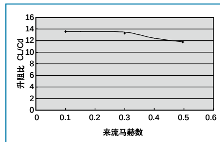
图7 迎角为 5^\circ 时升阻比与来流马赫数关系图
