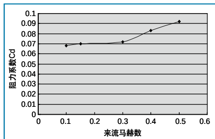
图6 迎角为 5^\circ 时阻力系数与来流马赫数关系图
