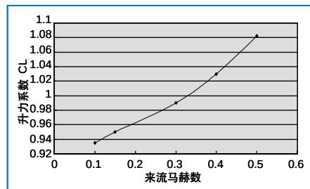
图5 迎角为 5^\circ 时升力系数与来流马赫数关系图
