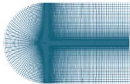
图1 机翼NACA5312网格划分图
