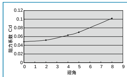
图3 马赫数为0.15时阻力系数与迎角关系图
